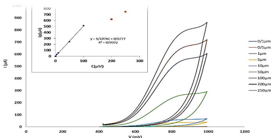
نمودار ۴- CV به‌دست آمده در غلظت‌های به‌دست آمده NIC از ۰/۱ تا ۱۰۰ میکرومولار
