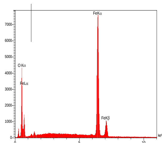
شکل ۴- آنالیز EDAX جاذب هیدروژل نانو مغناطیسی نشان‌دهنده وجود نانوذرات مغناطیسی آهن جهت جذب
