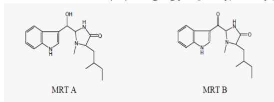
تصویر-۳. ساختار مارتنسنین A و B
