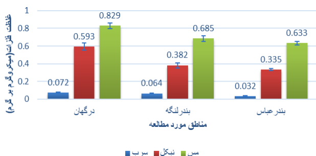
نمودار ۱-۱. مقایسه عناصر سرب، نیکل و مس در عضله ماهی شعری در مناطق درگهان، بندرخمیر و بندرعباس
