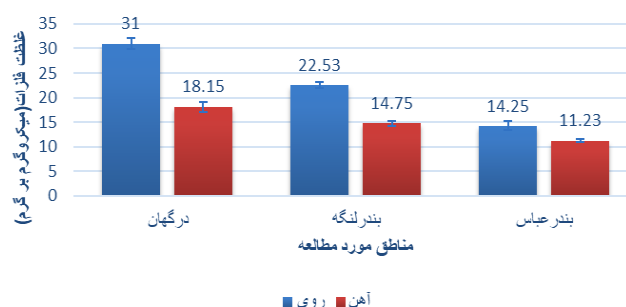
نمودار ۲-۲. مقایسه عناصر آهن و روی در عضله ماهی شعری در مناطق درگهان، بندرخمیر و بندرعباس
