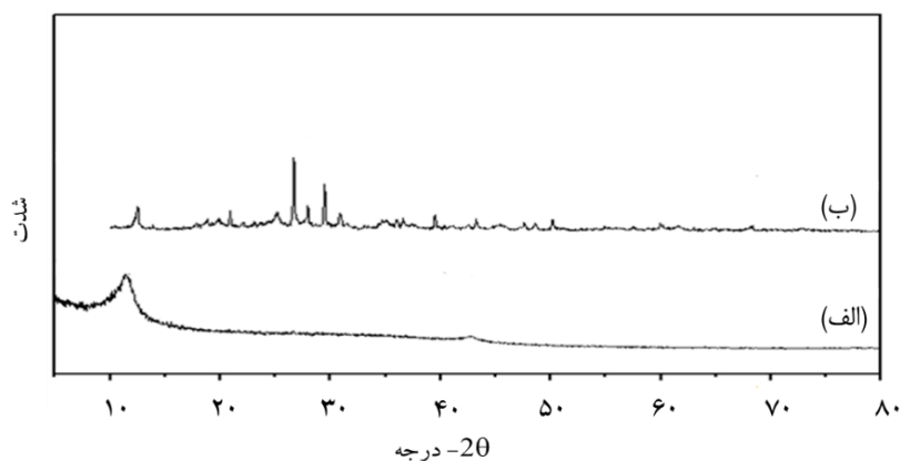
شکل-۱. مقایسه الگوی پراش پرتو ایکس (XRD) مربوط به نمونه‌های (الف) اکسیدگرافن (ب) اکسیدگرافن احیا شده با ماکروجلیک سبز
