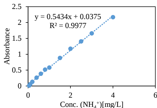
شکل ۱- نمودار کالیبراسیون جذب یون \text{NH}_4^+ دستگاه اسپکتروفتومتر UV در طول موج ۲۱۳ نانومتر
